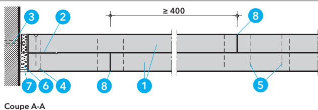
Coupe A-A
