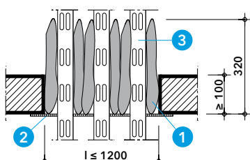
Coupe A-A
