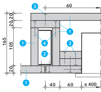
Querschnitt
