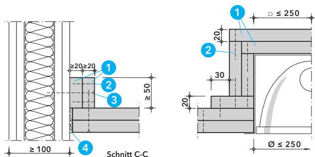
Schnitt C-C
