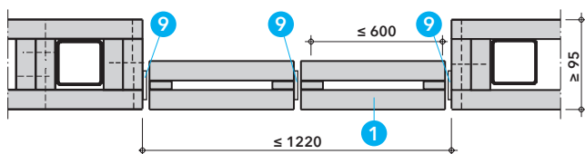
Schnitt H-H
