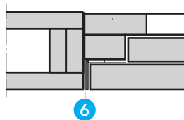
Schnitt E-E - Band- und Schlossseite
