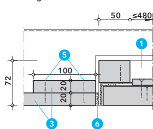
Längsschnitt
