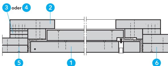
Revisionsklappe Promat®-Universal, Typ D
