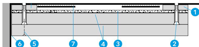
Alternativ Toison Promat® sûr les bandes PROMATECT®-XS
