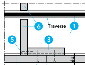
Section transversale \geq 600 mm coupe horizontale
