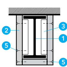
sans doublure horizontale du raccord, coupe verticale
