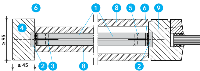
Paneel EI 60
