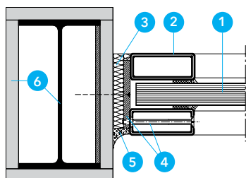
Eckausbildungen EI 60
