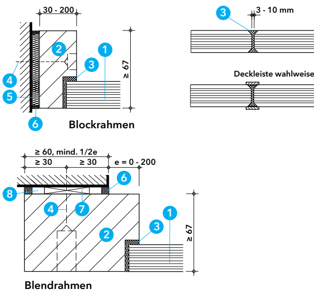
Blendrahmen
