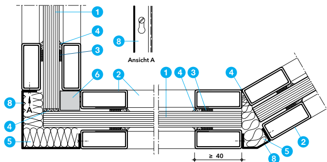
Eckausbildungen EI 60
