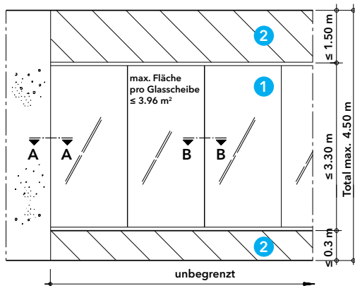
flächenbündig
