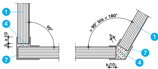
Eckausbildungen EI 30
