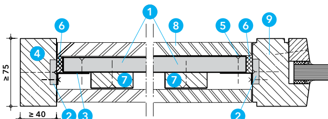
Paneel EI 30
