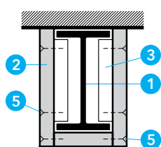
ohne waagrechter Stosshinterlegung Vertikalschnitt
