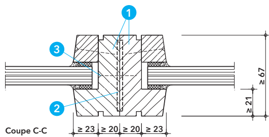
Coupe C-C
