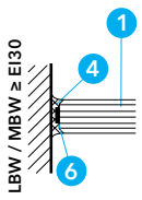
Variante: Stumpf
