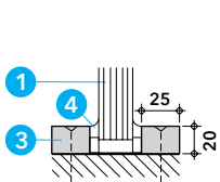
Variante: Glasleiste
