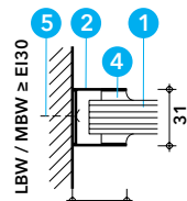
Variante: U-Profil nur mit Promat-SYSTEMGLAS 30, Typ 1-0
