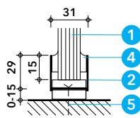
Variante: U-Profil nur mit Promat-SYSTEMGLAS 30, Typ 1-0
