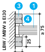
Variante: Glasleiste
