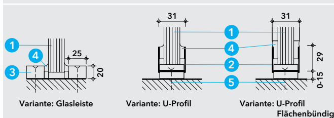
Detail B - Boden-/Deckenanschluss Schnitt C-C
