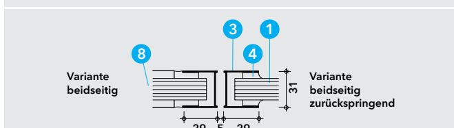
Detail D - Kombinationen mit Promat-Glastüren
