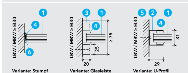
Detail A - Wandanschluss Schnitt A-A
