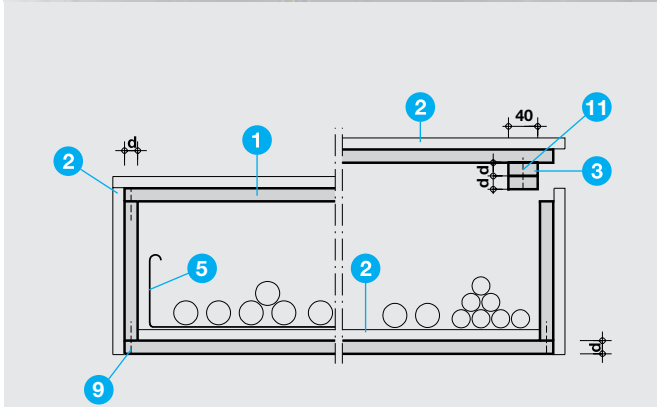
Detail A - Querschnitt
