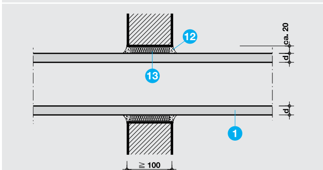
Detail D - Wanddurchführung
